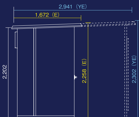
《側面図》
